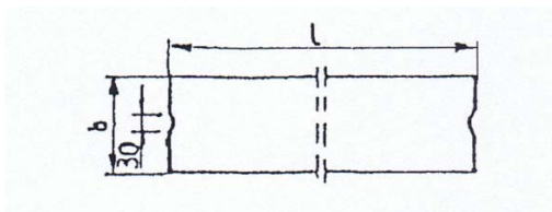
Rys. 1. Wymiarowanie krawężników
